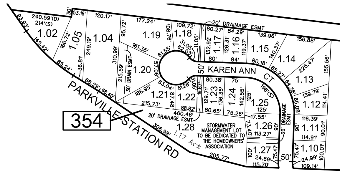
DETAIL "A" SCALE: 1" = 200'
